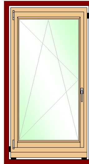
Beispiel. Anordnung der Tragklötze bei einem Dreh-Kipp-Fenster
