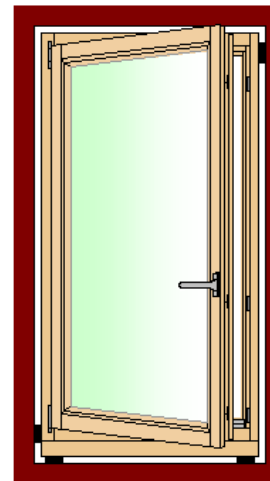
Beispiel. Anordnung der Tragklötze bei einem Dreh-Kipp-Fenster
